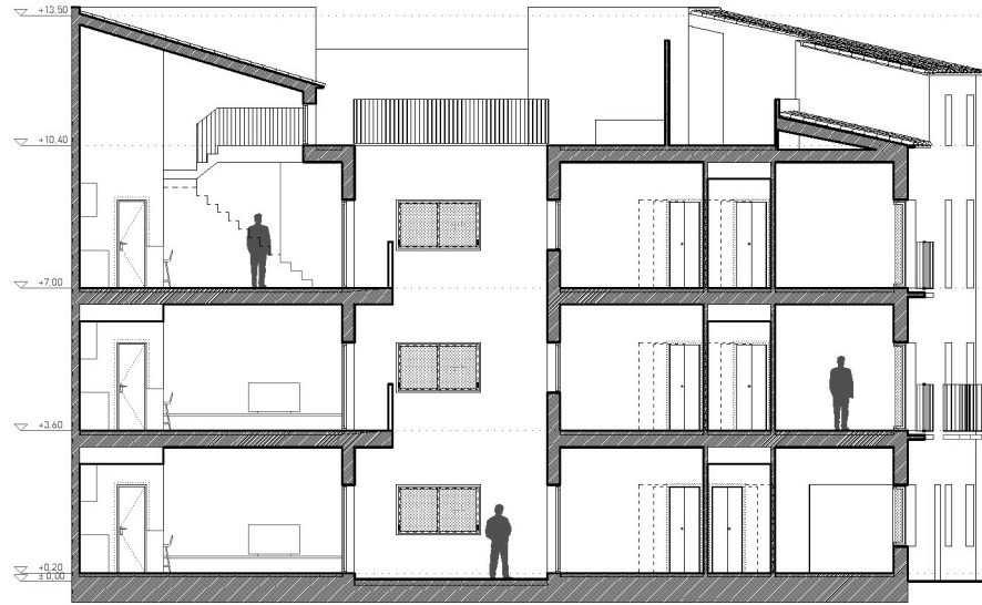
Sección 2
