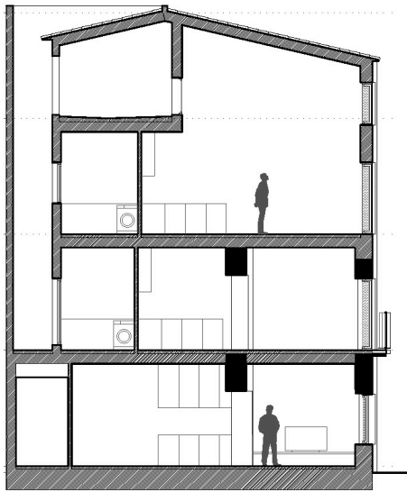
Sección 1
