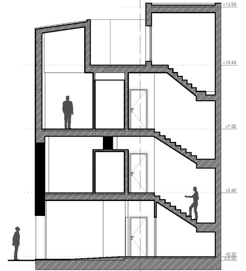
Sección 3
